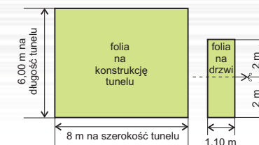
Schemat 5 MONTAŻ FOLII
