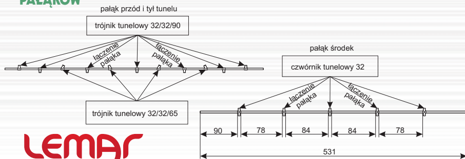
Schemat 2 MONTAŻ PAŁKÓW
