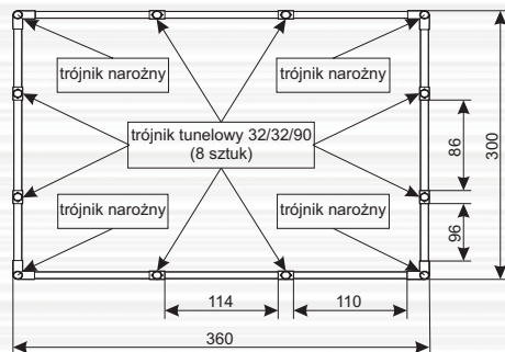
Schemat 1 MONTAŻ RAMY TUNELU
