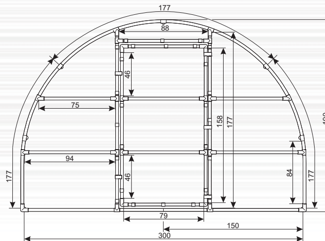
Schemat 3 MONTAŻ DRZWI TUNELU
